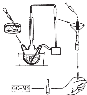
图 2 蒸馏吸附分析法
