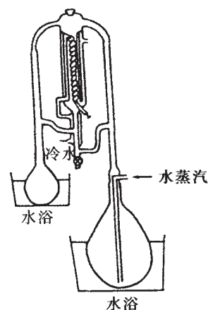
图 1 连续蒸馏萃取法
